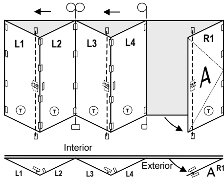
4L1RSOFD1DG
