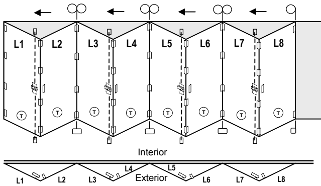
8LSOFD1DG
