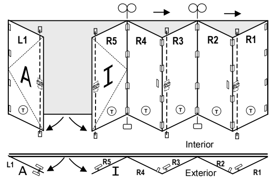
1L5RSOFD1DG
