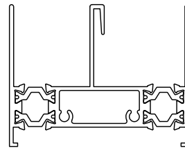
#1251 JAMB
